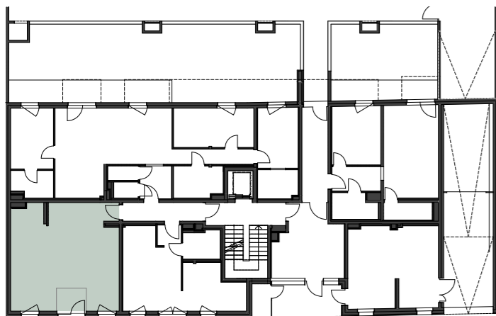
ÜBERSICHTSPLAN ERDRGESCHOSS
