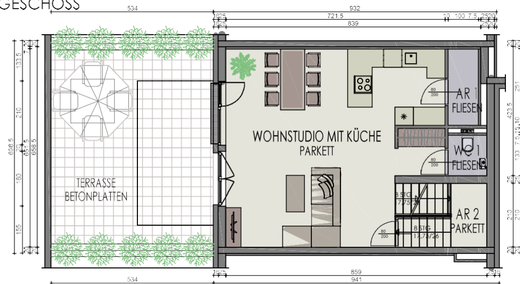
GARTENGESCHOSS
