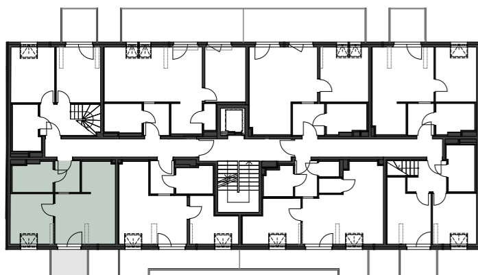
ÜBERSICHTSPLAN 1. DACHGESCHOSS
